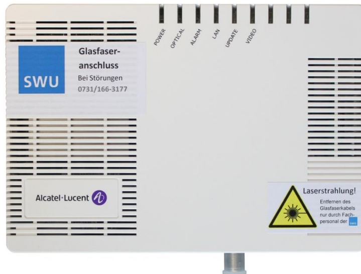
SFU Frontansicht
